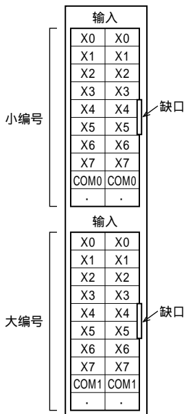
FX5-C32EX/DS
