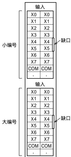
FX5-C32EX/D
