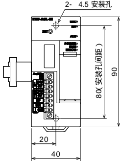
FX5-ASL-M
