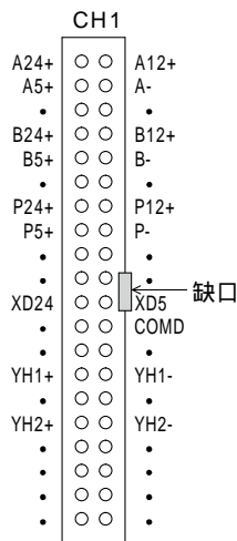
FX3U-2HC
