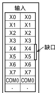
FX5-C16EX/DS
