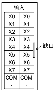
FX5-C16EX/D
