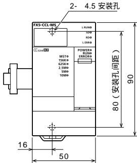
FX5-CCL-MS
